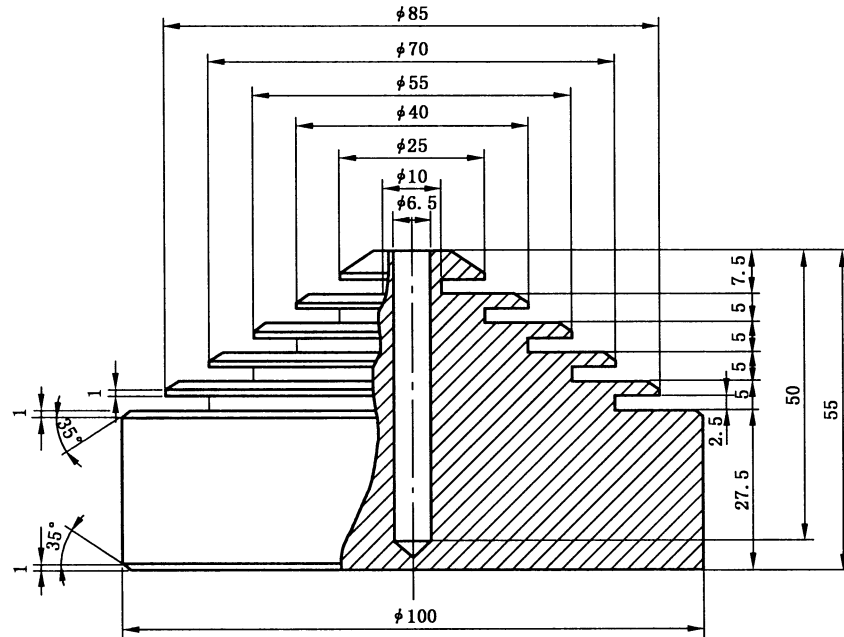
图1 热源块
